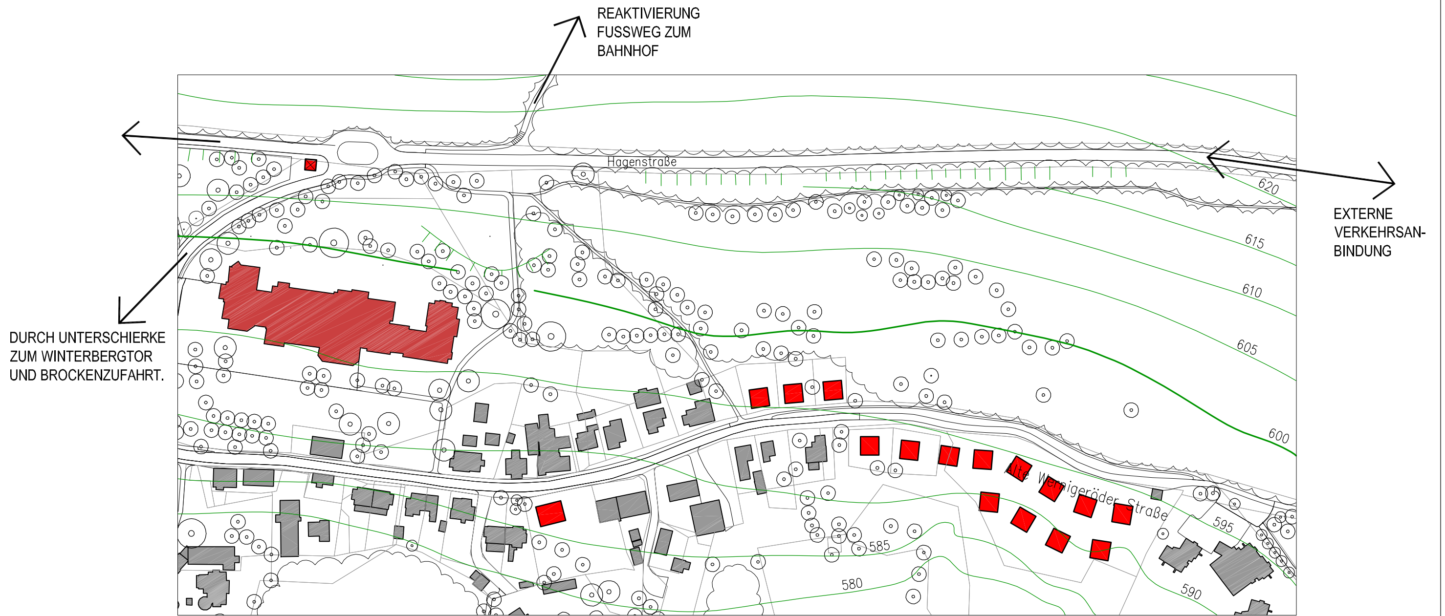
ÜBERSICHT M 1:2000
