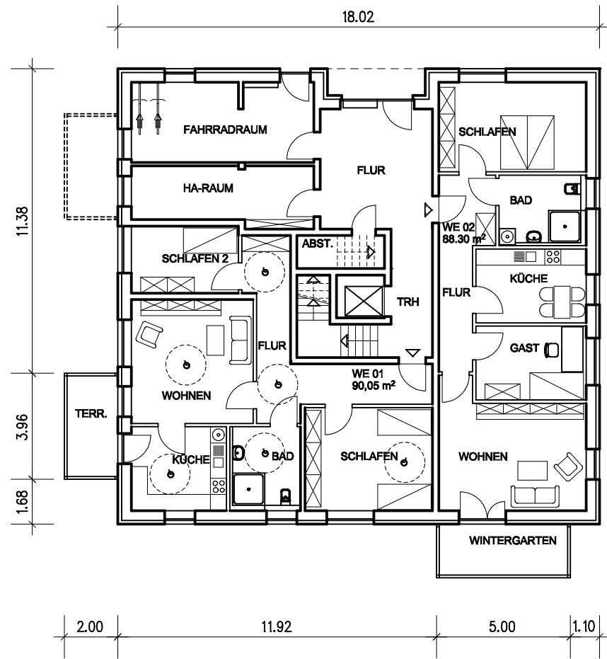
NORMALGESCHOSS
