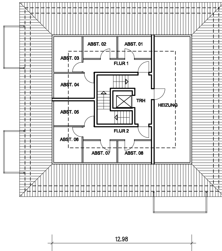
DACHGESCHOSS
