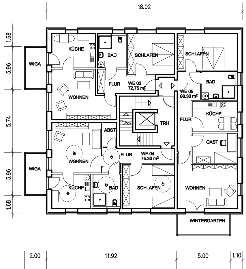
NORMALGESCHOSS
