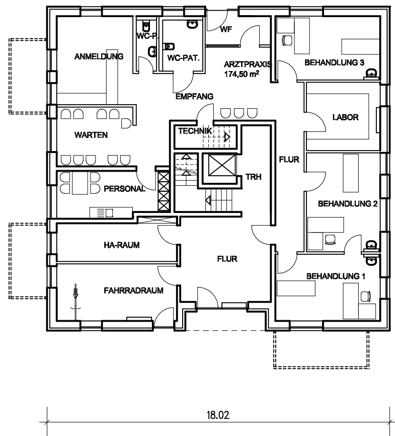
ERDGESCHOSS GERWERBE
