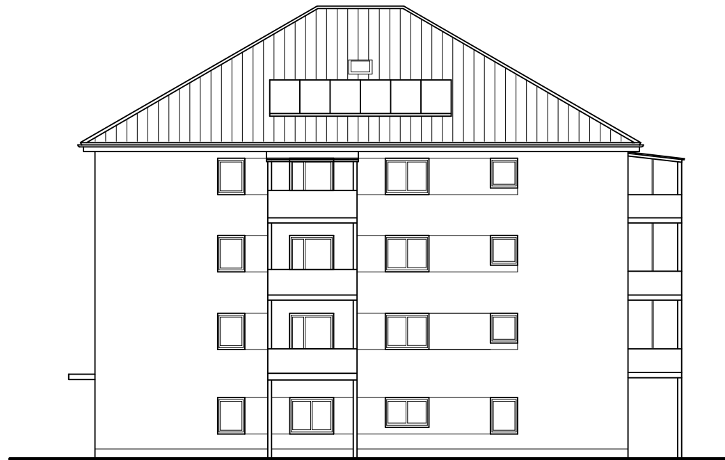
ANSICHT SÜDOST
